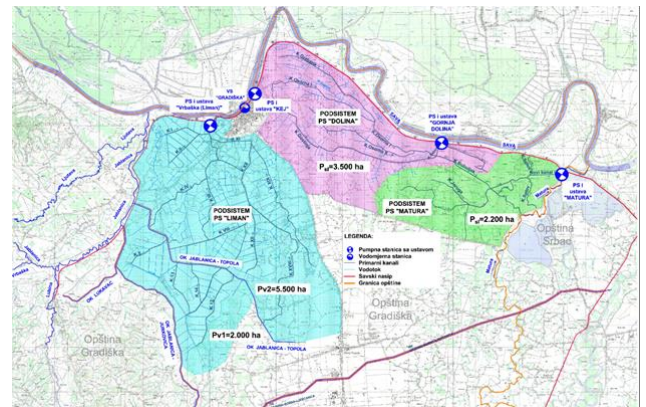
Прегледна карта подсистема одводње
