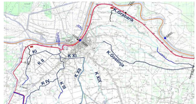
Прегледна карта канала
