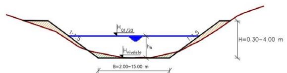
Карактеристични попречни профил канала
